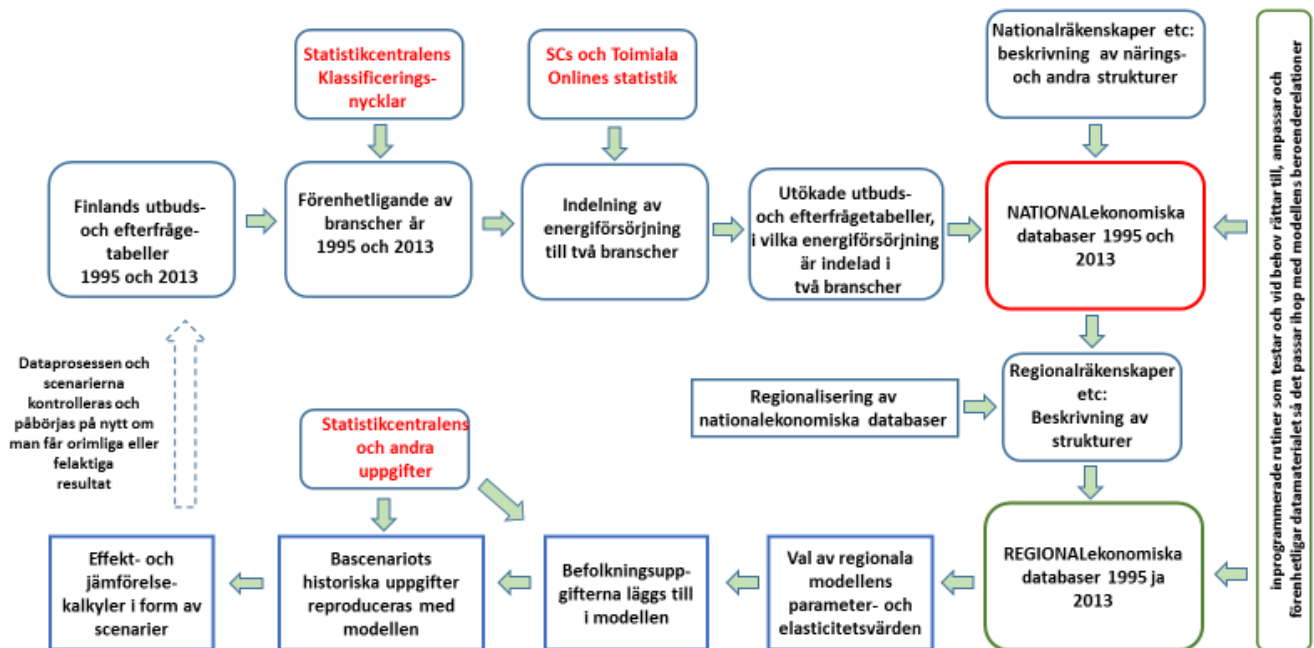
Figur 12. Beskrivning av uppbyggnaden av grunddata och analysen i RegFinDyn.
