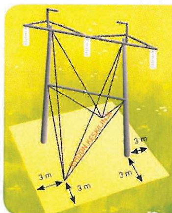
Harustettu, kaksijalkainen pylväs
